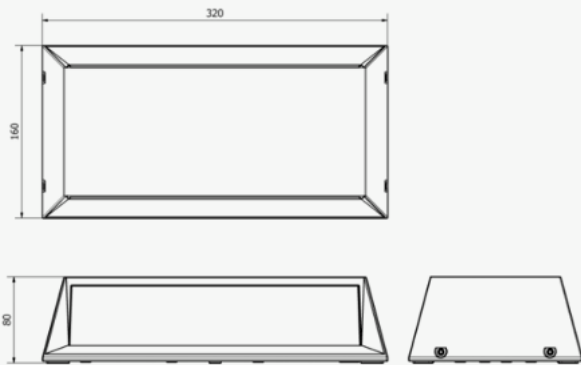
Schutzwanne SYMM Plus (Abmessungen in mm)
