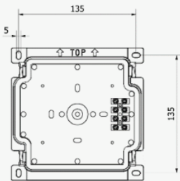
Montageplatte SYMM (Abmessungen in mm)
