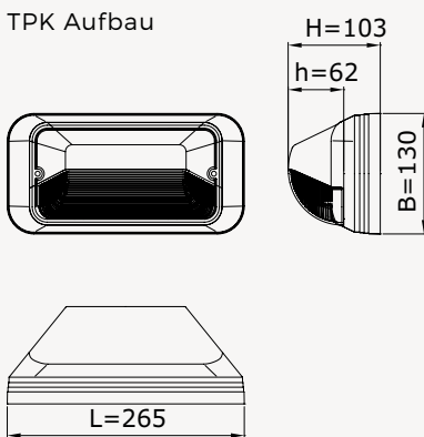
TPK Aufbau
